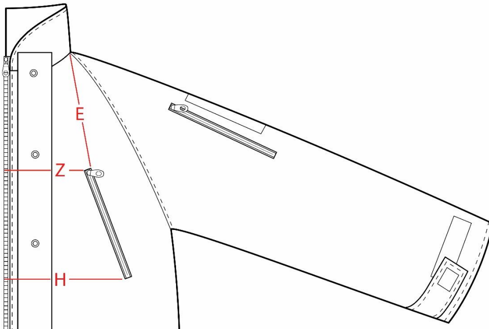
Σχέδιο 3. Σημεία μέτρησης τσέπης εμπρόσθιου τμήματος κορμού επενδύτη
