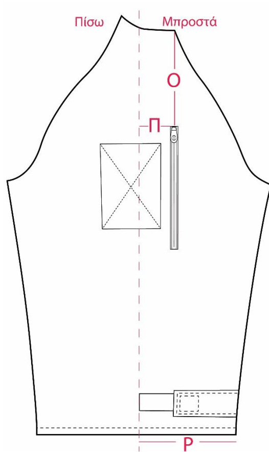
Σχέδιο 10. Σημεία μέτρησης μανικιού
