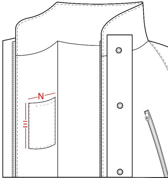
Σχέδιο 9. Σημεία μέτρησης εσωτερικής τσέπης κορμού
