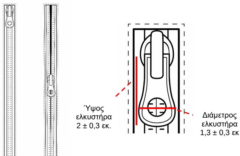
Σχέδιο 1. Πλαστικό διαχωριζόμενο φερμουάρ, με εσωτερικά δόντια
