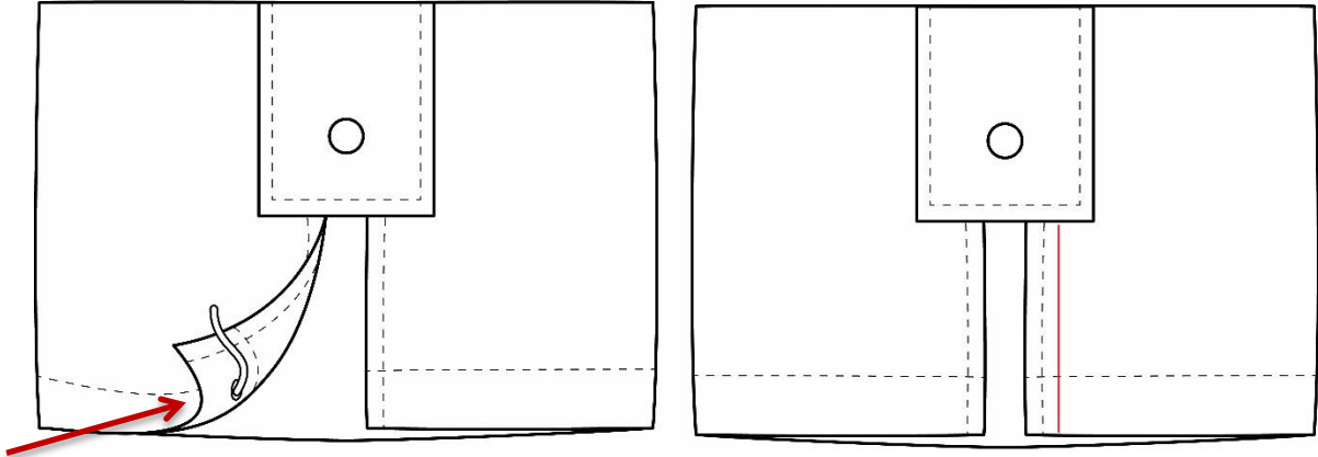
Σχέδιο 8. Τελείωμα ρούχα (παράγραφος 4.3.2.2.1)
