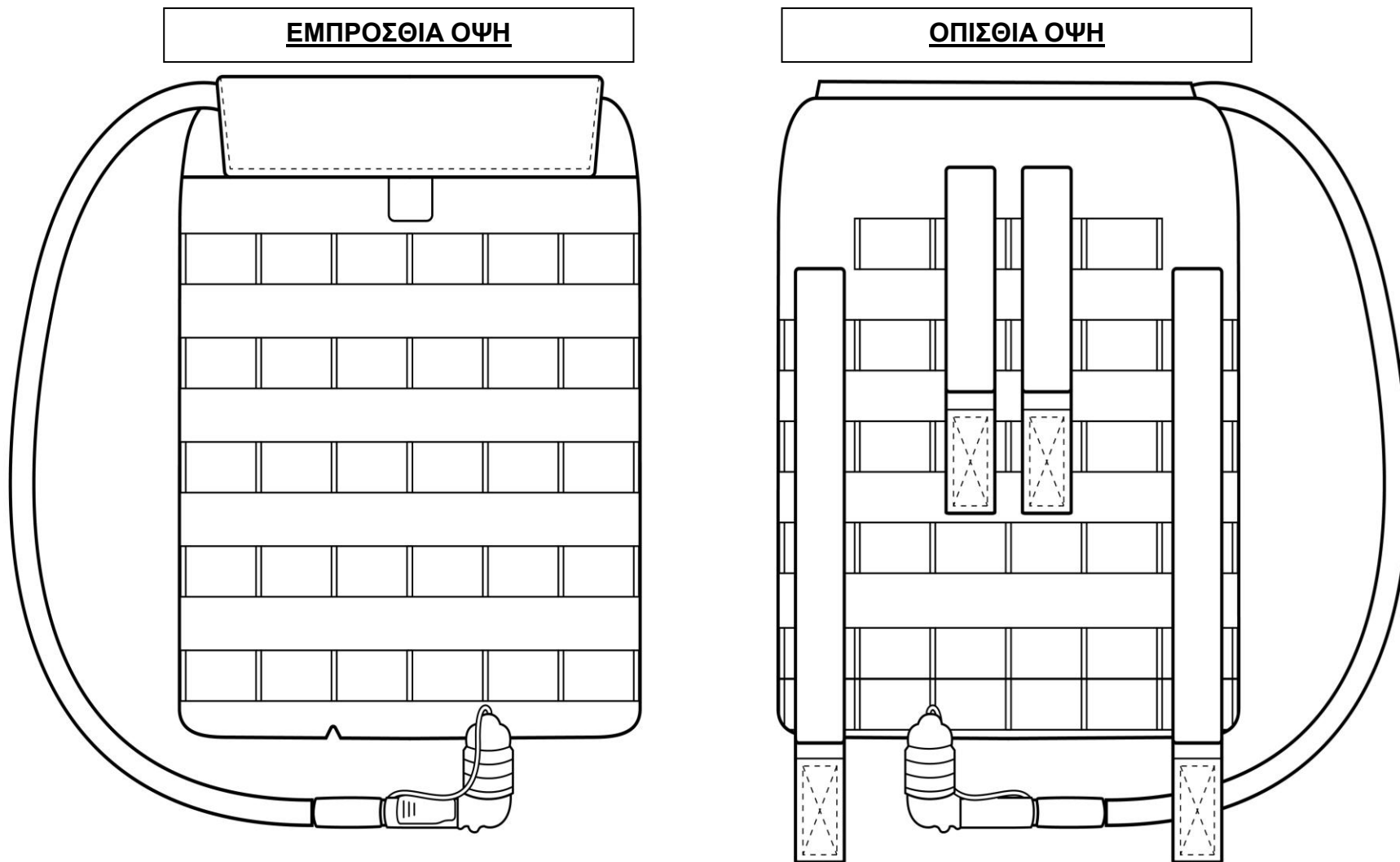
Εικόνα 15. Κατασκευαστικό Σχέδιο Υδροδοχείου Πλάτης
