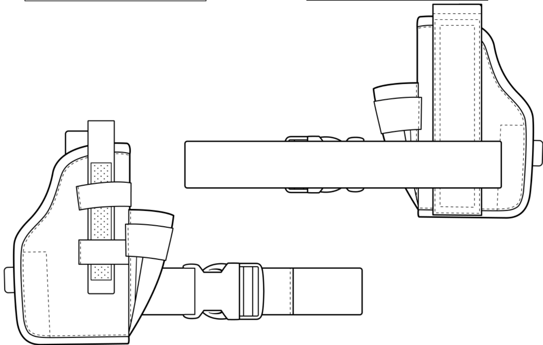
Εικόνα 23. Κατασκευαστικό Σχέδιο Πιστολοθήκης με Θήκη Γεμιστήρα
