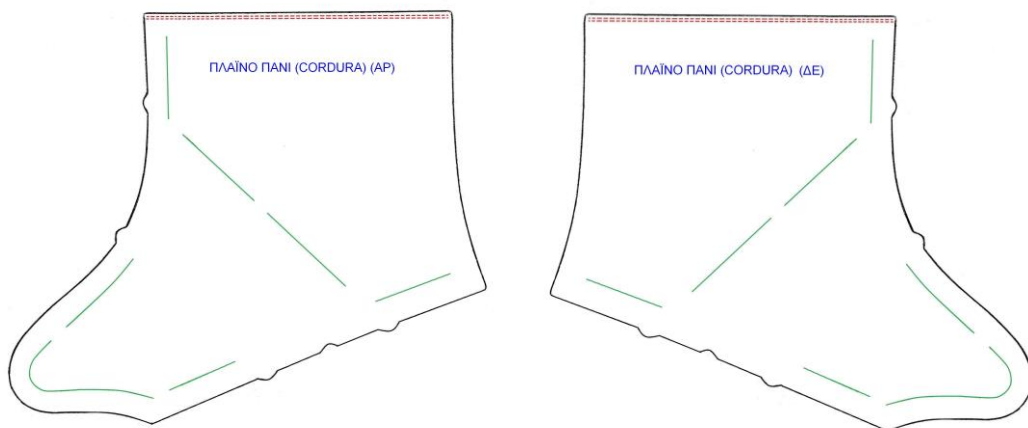
Εικόνα 4: Σχέδιο Πλαϊνά (ΑΡ – ΔΕ) από ύφασμα cordura
