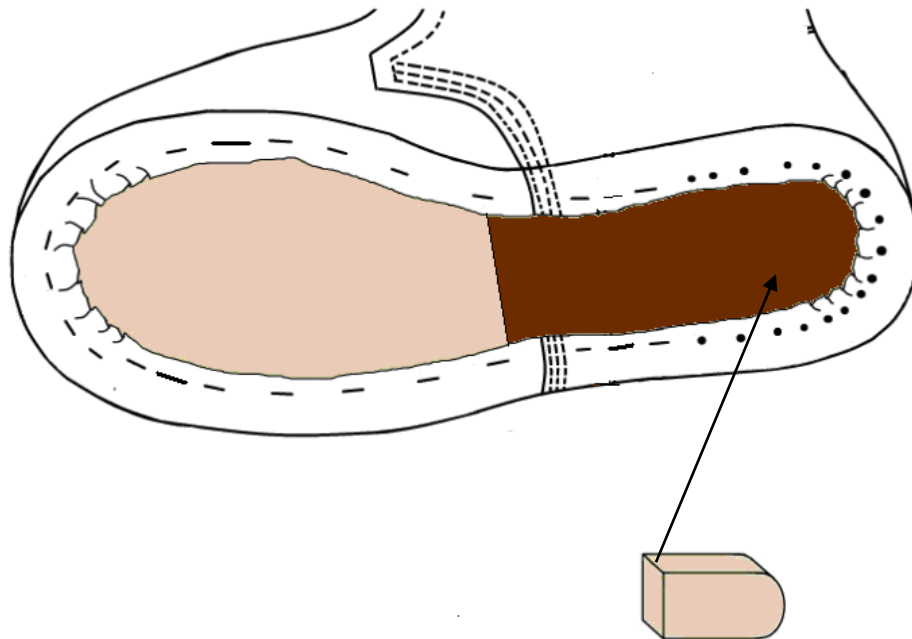
Σχ.6 Κάτω όψη φοντίου μονταρισμένου (πριν τον βουλκανισμό) και πληρωτικό τακουινιού
